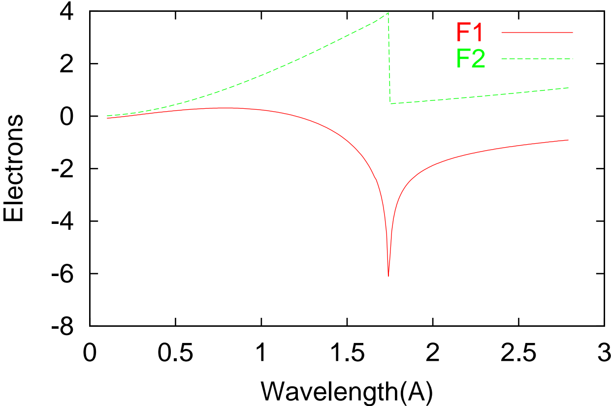
Absorption Data ( FE.WIDE )
