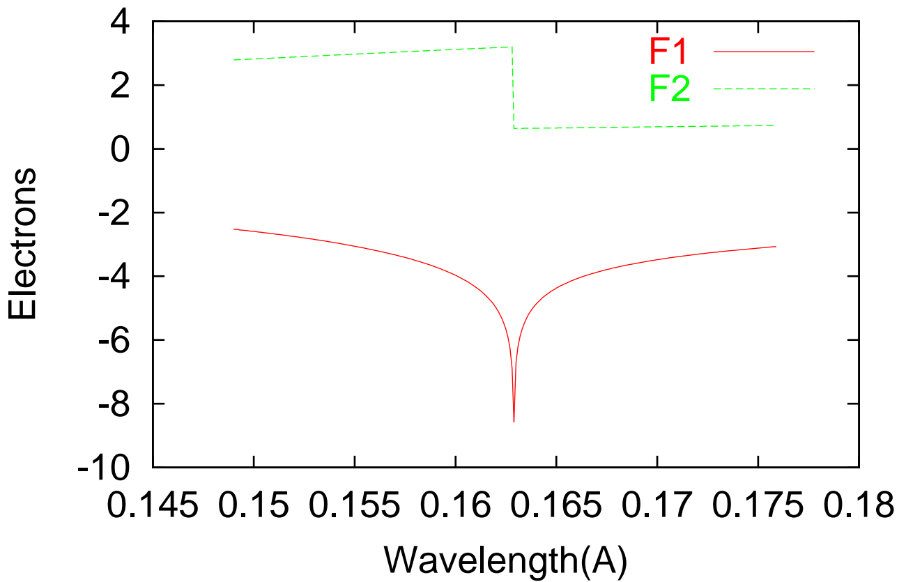
Absorption Data IR.K
